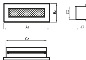
Kratka - czerpnia KRCZNP 150x50, 200x50 i 200x90
