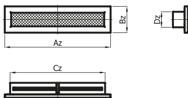
Kratka - czerpnia KRCZNP 300x50
