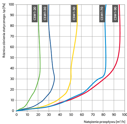
Wykres strat ciśnienia stabilizatorów w zależności od natężenia przepływającego powietrza.
