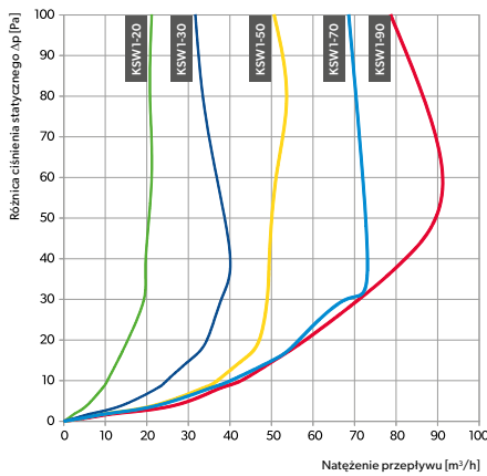
Wykres strat ciśnienia stabilizatorów w zależności od natężenia przepływającego powietrza.
