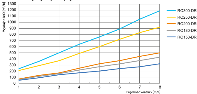
Wykres wydajności samonastawnych nasad kominowych ROTOWENT DRAGON w zależności od prędkości wiejącego wiatru bez uwzględnienia wysokości kominu. *1 [m/s] = 3.6 [km/h]
