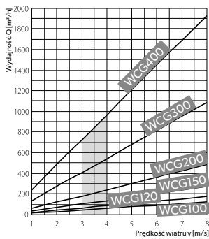
Wykres wydajności wywietrzaków cylindrycznych (CAG) w zależności od prędkości wiejącego wiatru bez uwzględnienia wysokości kominu. *1 [m/s] = 3.6 [km/h]
