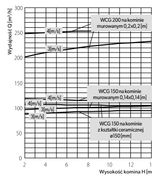
Wykres wydajności wywietrzaków cylindrycznych ø200, 150 dla komin blaszanych i murowanych, dla dwóch prędkości wiatru 3 i 4 [m/s].
