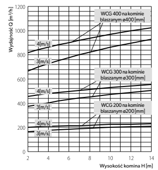
Wykres wydajności wywietrzaków cylindrycznych ø200, 300, 400 dla komin blaszanych, dla dwóch prędkości wiatru 3 i 4 [m/s].
