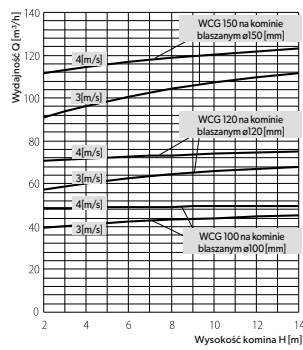
Wykres wydajności wywietrzaków cylindrycznych ø100, 120, 150 dla komin blaszanych, dla dwóch prędkości wiatru 3 i 4 [m/s].
