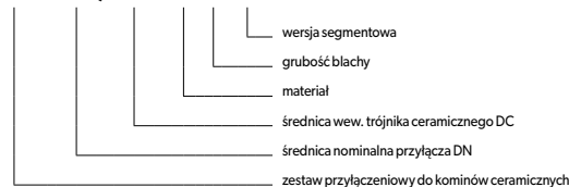
WKC-S
