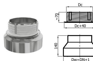
WKC-S
